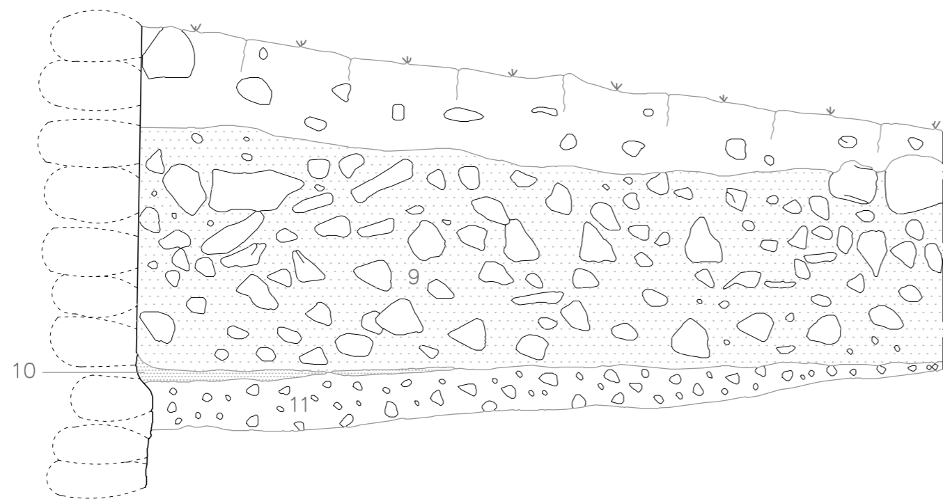
Saggio 1 - sezione est
