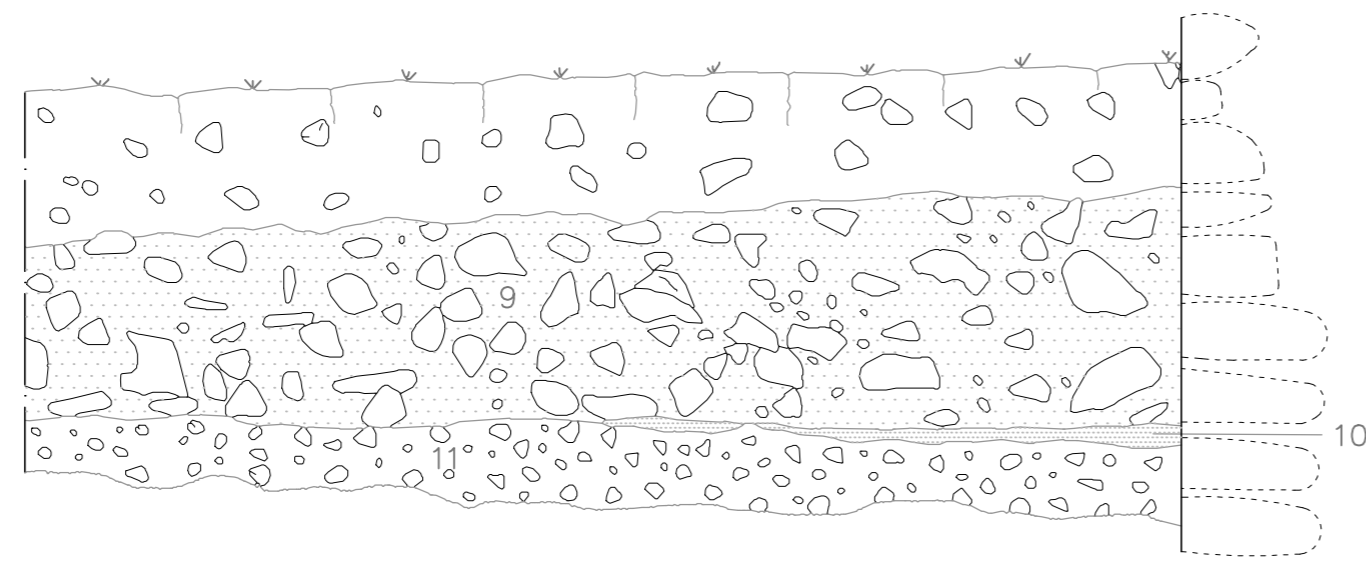
Saggio 1 - sezione ovest
